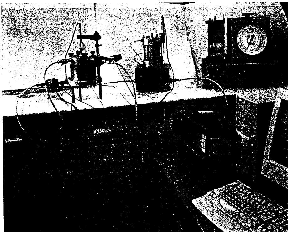
شکل شماره ۳ - نمای کلی دستگاه تحکیم هیدرولیکی و تجهیزات ضمیمه (۱- دستگاه تحکیم هیدرولیکی ۲- دستگاه تعیین حجم ۳- دستگاه مولد فشار ۴- دیتالاگر)
